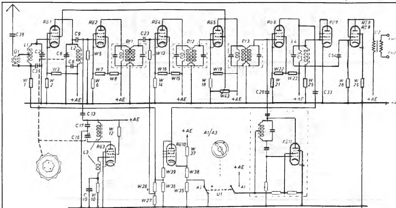
OBR.8: Zjednodušené schéma krátkovlnného prijímače E10OaK. U1 prispôsobovací v'f transformátor. R01 ladený vstupný zesilovač, R03 oscilátor, R02 smesovač, R04, R05 a R06 trístupňový MF zesilovač - medzi MF transformátory - trimry /nejsou zakresleny/. R07 je an. didový detektor, R08 a R09 je zdvojený nf zesilovač. FH1 a FH2 jsou vývody pro sluchátka. R010 je stupeň řídicího napětí AVC. R011 je BFO. W43 řízení hlasitosti změnou napětí stínících mřížek R01 a R05. C2, C8 a C16 je ladící kondenzátor - triál.
