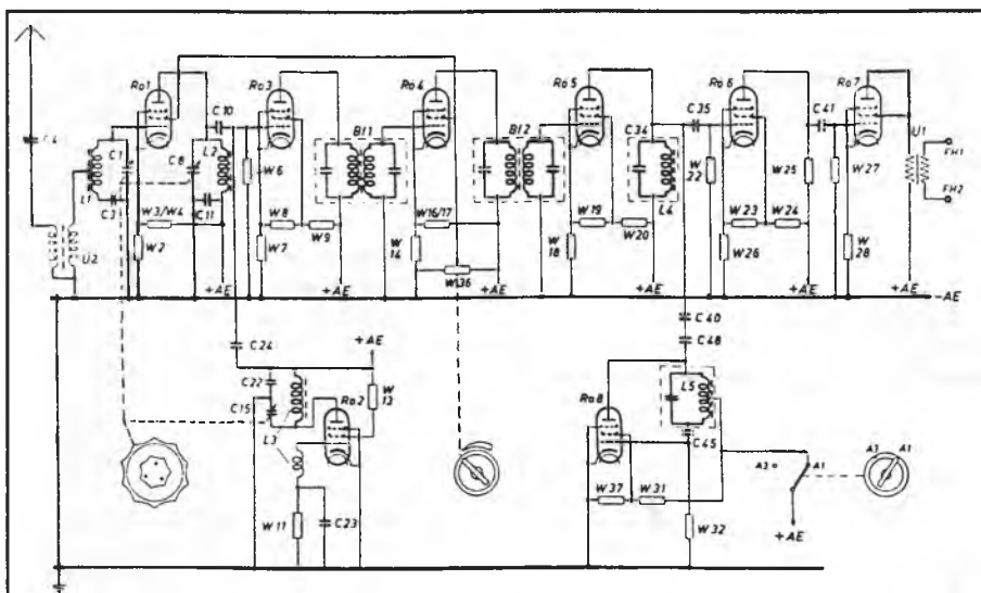
OBR.7: Zjednodušené schéma krátkovlnného prijímače E10K. U2 - impedanci antény prispôsobujúci v'f transformátor. R01 ladený vstupný v'f zesilovač, R02 oscilátor, R03, R04 a R05 dvoustupňový MF zesilovač s kapacitní vazbou /nezakresleno/. R06 anodový detektor, R08 BFO, R07 nf zesilovač s výstupným transformátorem. W36 nastavení hlasitosti změnou napětí stínících mřížek R01 a R04. C1, C8 a C15 ladící kondenzátor - triál.
