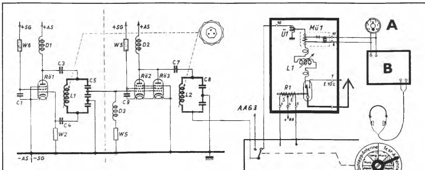
OBR.3: Základní schéma dlouhovlnného vysílače S10L a S10 a anténního přístroje AAG2. Rol - třibodový oscilátor, L1 a L2 - duál ladících indukčností - ladění jemně, W5 odpor představující dělič mřížkového předpětí umístěný v ovládací skříňce FBG3. Ro2 a Ro3 zdvojený koncový stupeň. Anténní přístroj AAG2 vpravo: U1 impedanční přizpůsobení antény. Mü1 obvod pro měření anténního proudu, L1 dálkově ovládaný variometr vyladění antény, R1 vakuové relé vysílání / příjem. Přepínač v poloze „pevná dlouhovlnná anténa“. B je zesilovač poslechu. Vpravo dole je štítek přepínače v ovládacím přístroji FBG3.
