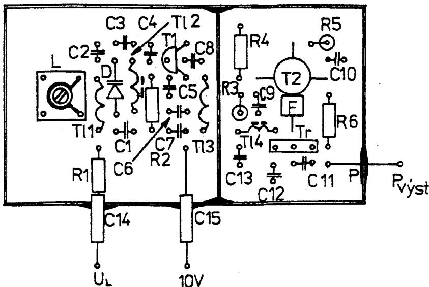
Obr.6 - Osazení plošného spoje (zvětšeno)
