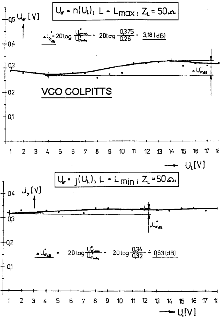
Obr.3 - Amplitudové charakteristiky VCO
