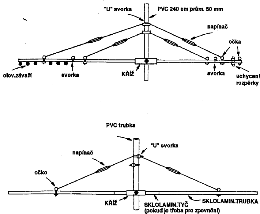
Obr.4 - Vytužení antény proti prohnutí
