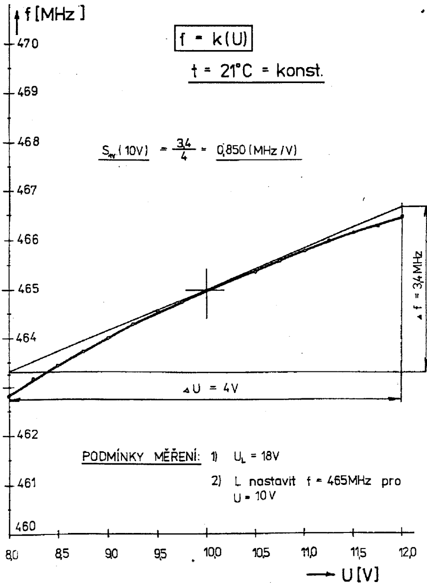
Obr.5 - Kmitočtová závislost VCO na napájení
