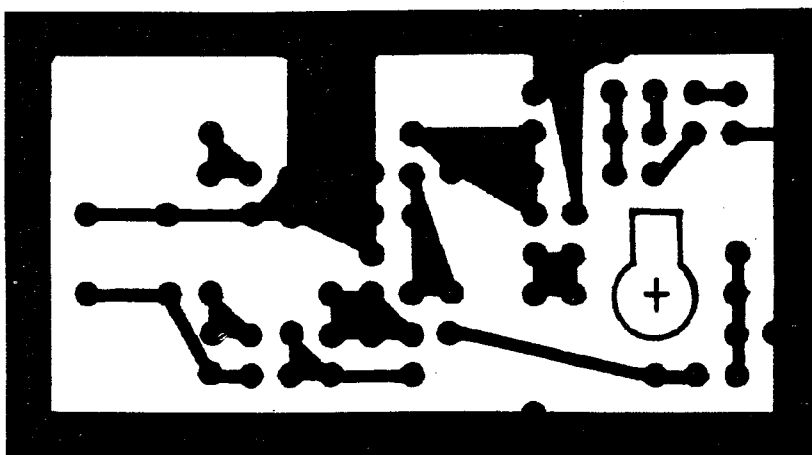
ROZMĚRY 50 x 27,5 mm materiál modrý sklotextil - jednostranný
