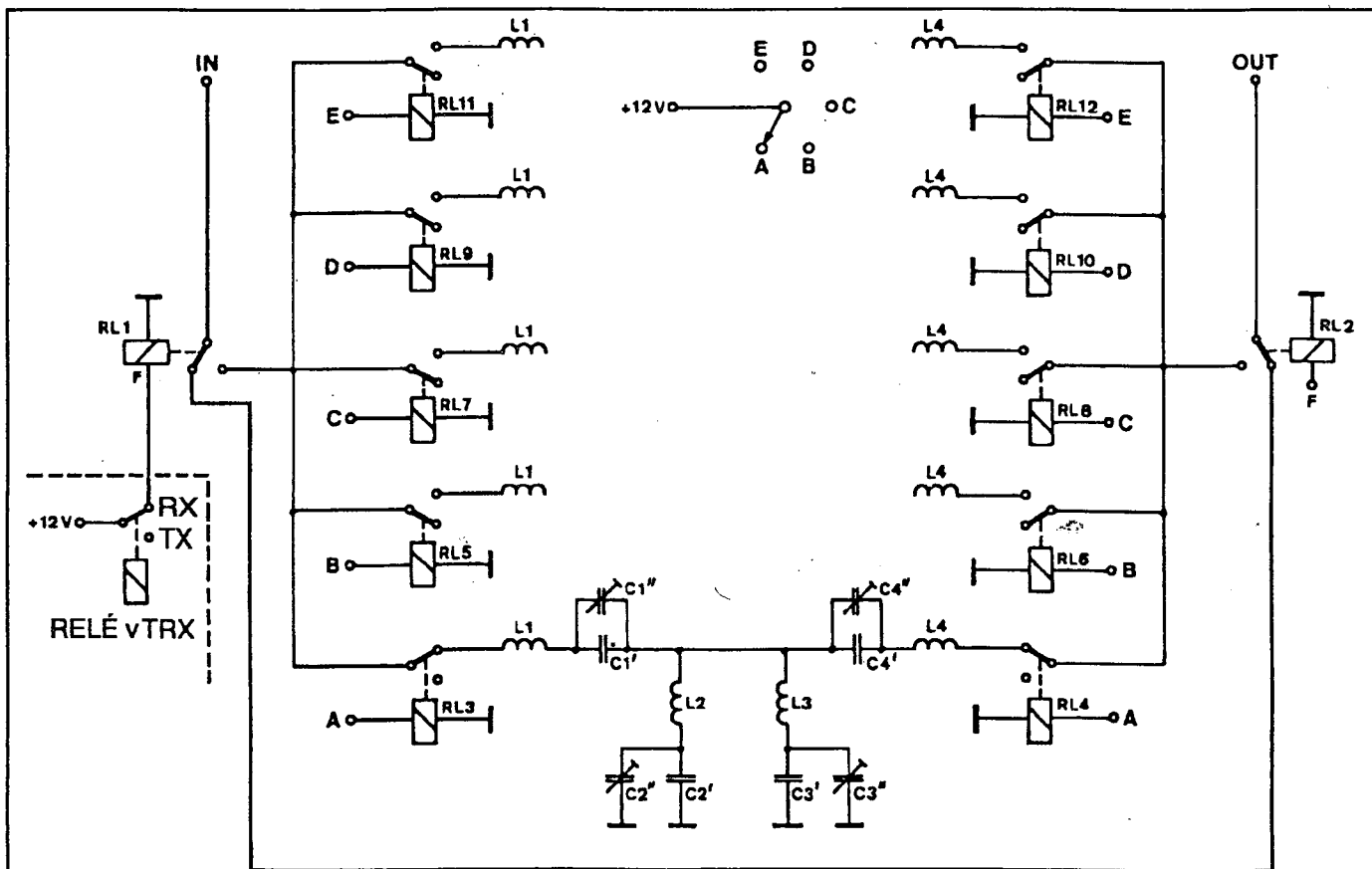
Obr.2 - Skutečné zapojení pásmových filtrů
