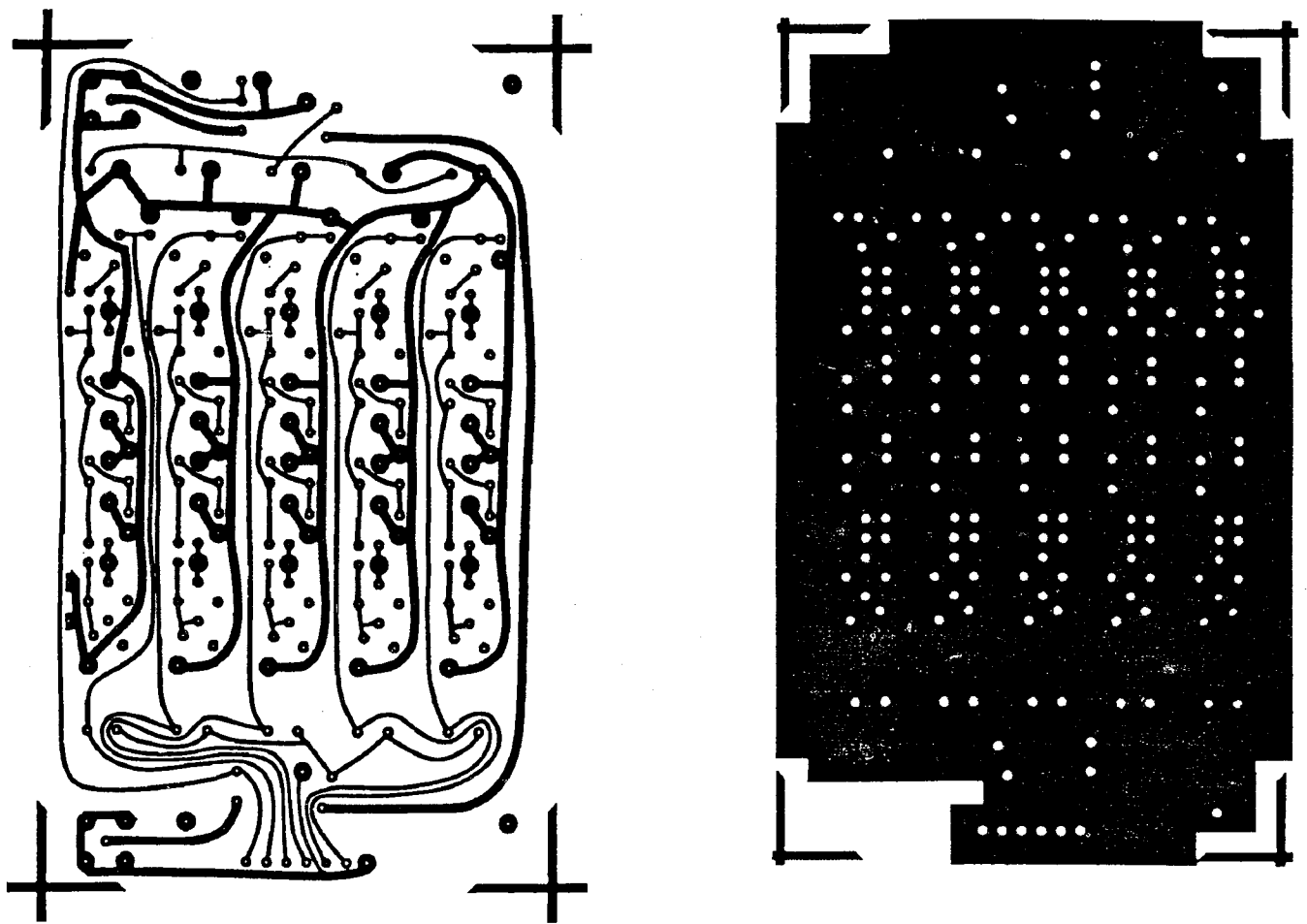
Obr.3 - Tištěný spoj ze strany spojů (vlevo) a součástek (vpravo)
