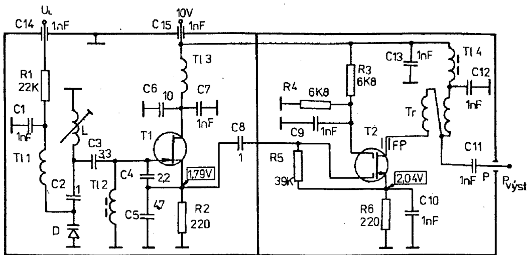
Obr.1 - Zapojení VCO
