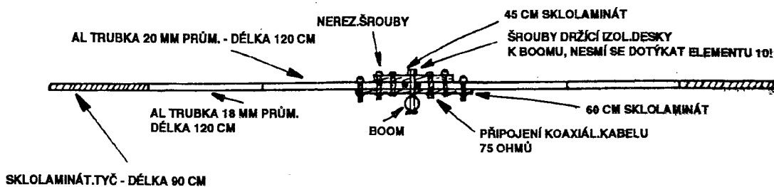
Obr.3 - Podrobný náčrt prvku č.10 a jeho uchycení
